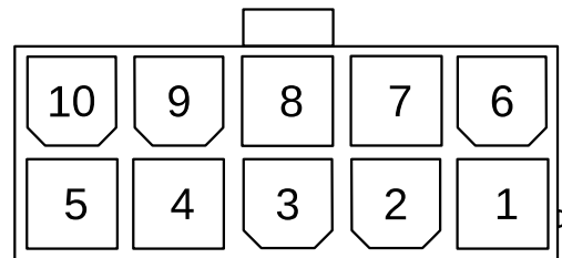
Ansicht des Steckers im Steuergerät
