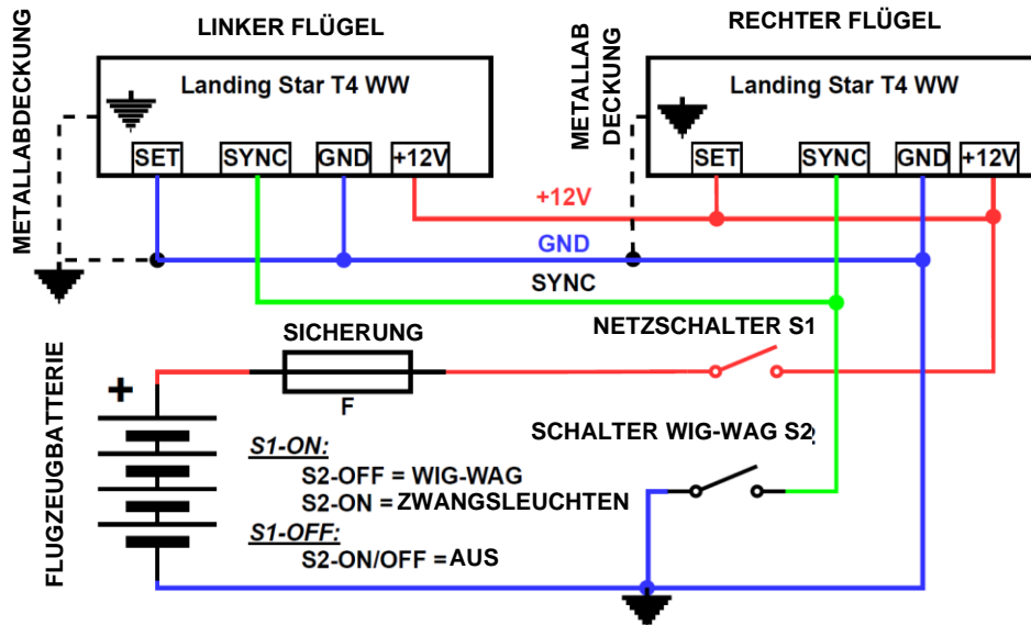
Abb. 3: Schaltplan für zwei Strahler
