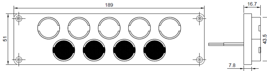
Abb. 1: Scheinwerferabmessungen
