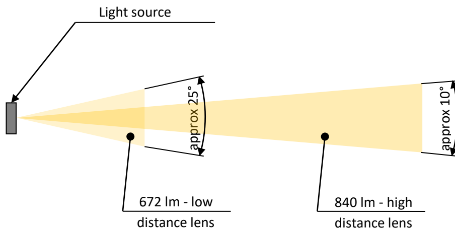
Abb. 4: Strahlungseigenschaften des Scheinwerfers
