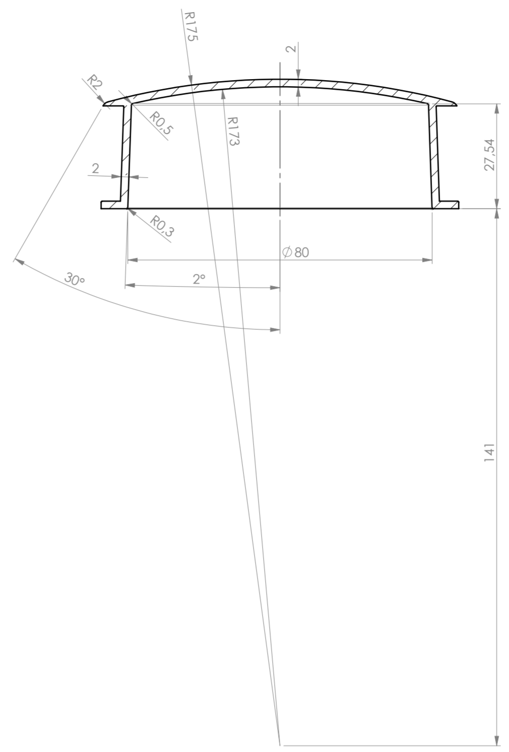
ŘEZ A-A
